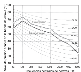
MMY-MUP1201HT8P-E Nivel de presión sonora (dB(A)) Refrigier. Calefacc. 58.0 62.0
