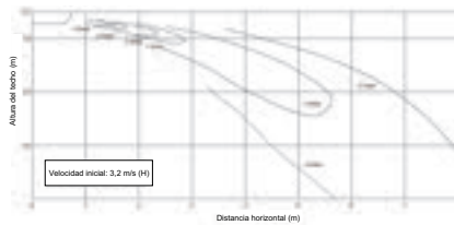
MMC-UP0561HP-E Refrigeración
