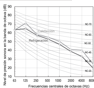
MMY-MUP1001HT8P-E Nivel de presión sonora (dB(A)) Refrigier. Calefacc. 55.0 58.0
